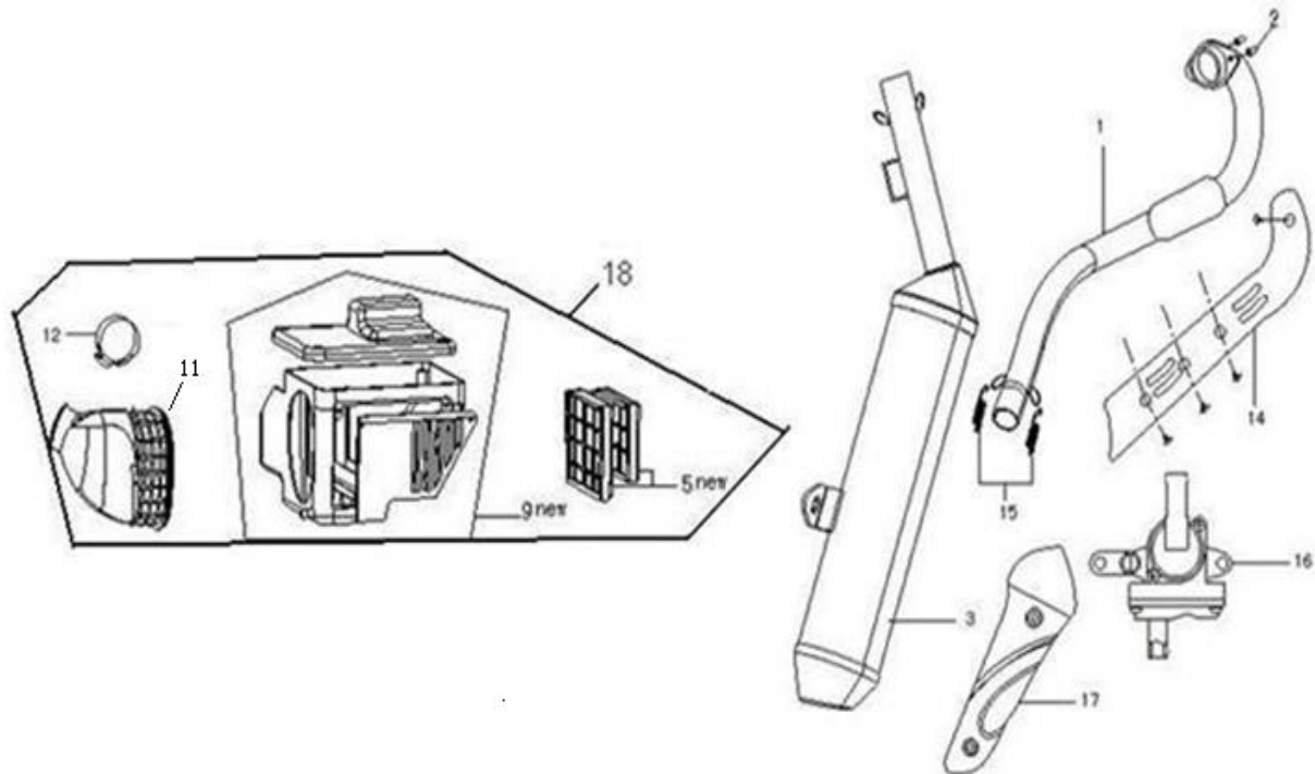
空滤器/排气消声器 AIR FILTER/MUFFLER
