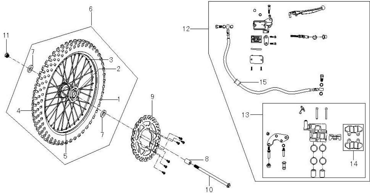
前轮/前碟刹 FR. WHEEL/FR. DISK BRAKE
