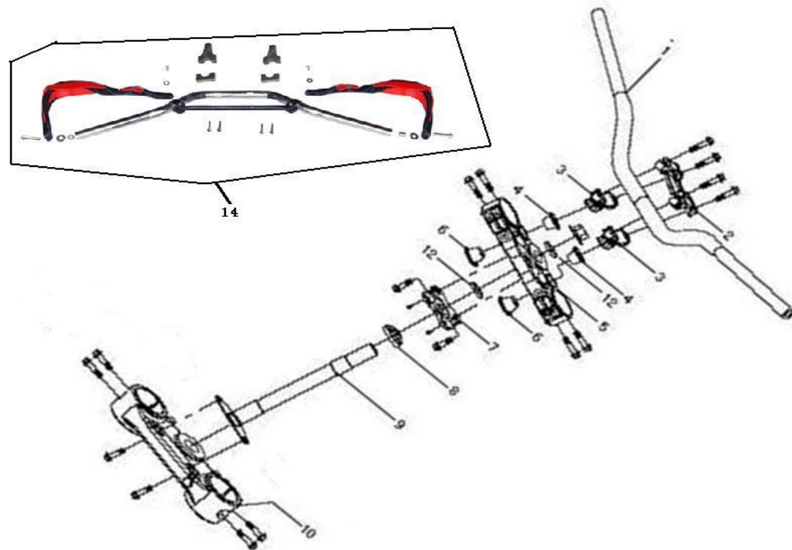
方向把/方向柱 HANDLE BAR/STEERING STEM
