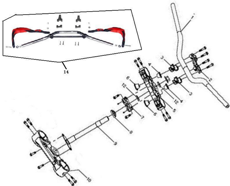
方向把/方向柱 HANDLE BAR/STEERING STEM
