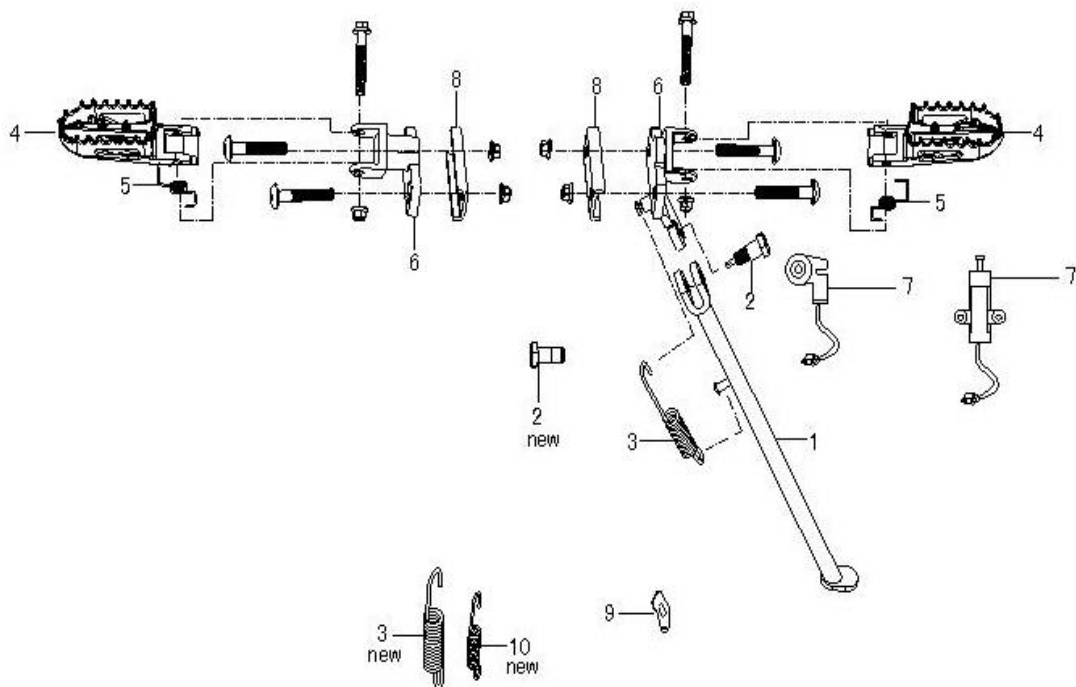
脚踏/侧支架 FOOT PEG/KICK STAND ASSY
