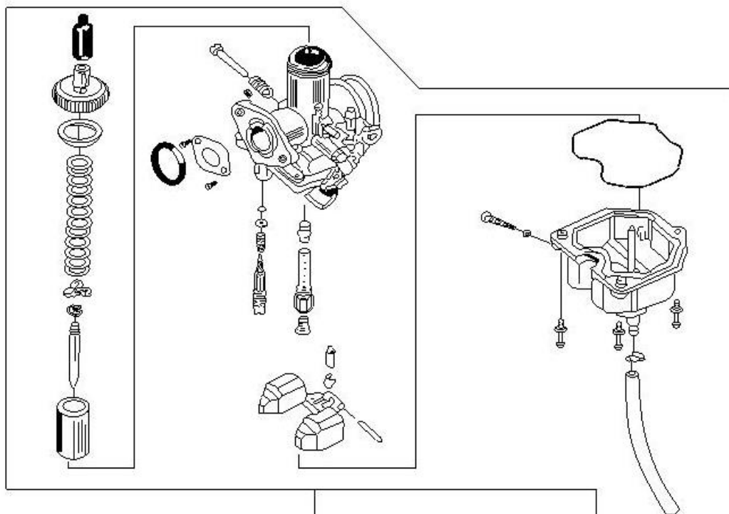
化油器 CARBURETOR
