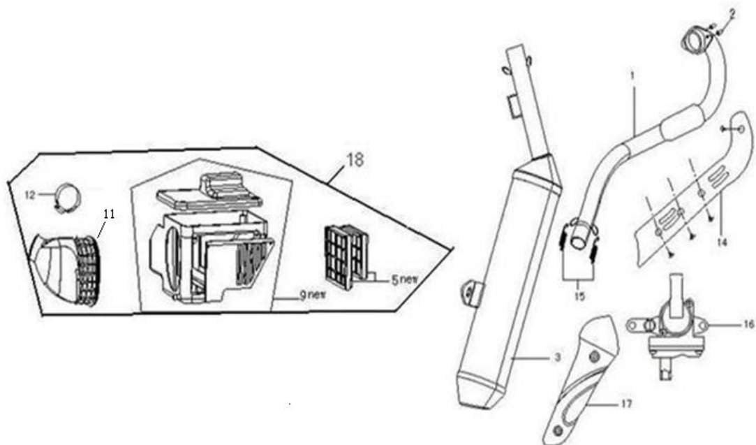
空滤器/排气消声器 AIR FILTER/MUFFLER
