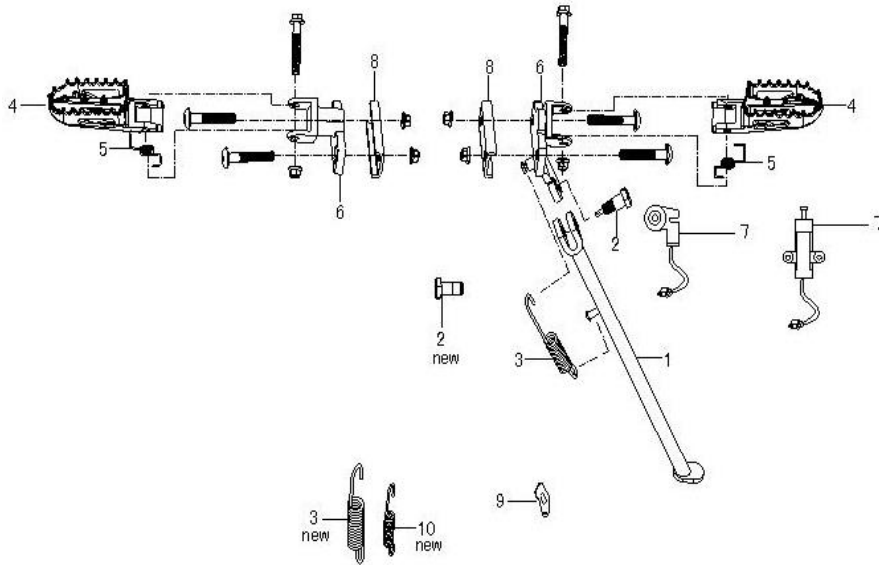
脚踏/侧支架 FOOT PEG/KICK STAND ASSY
